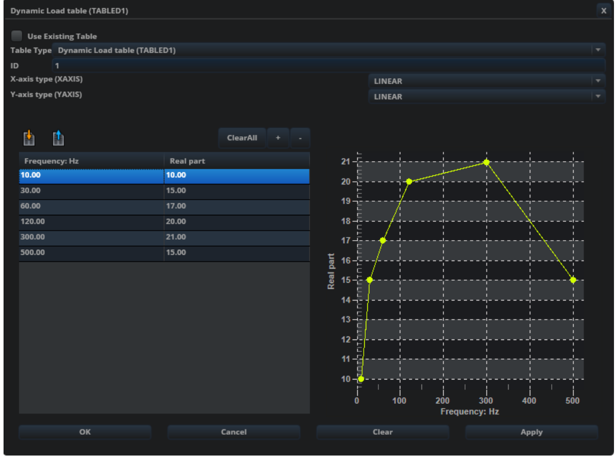
ŞEKİL 5 YÜKLERİN FREKANS BAĞLI GRAFİKLERİ İÇEREN TABLO ARACI
