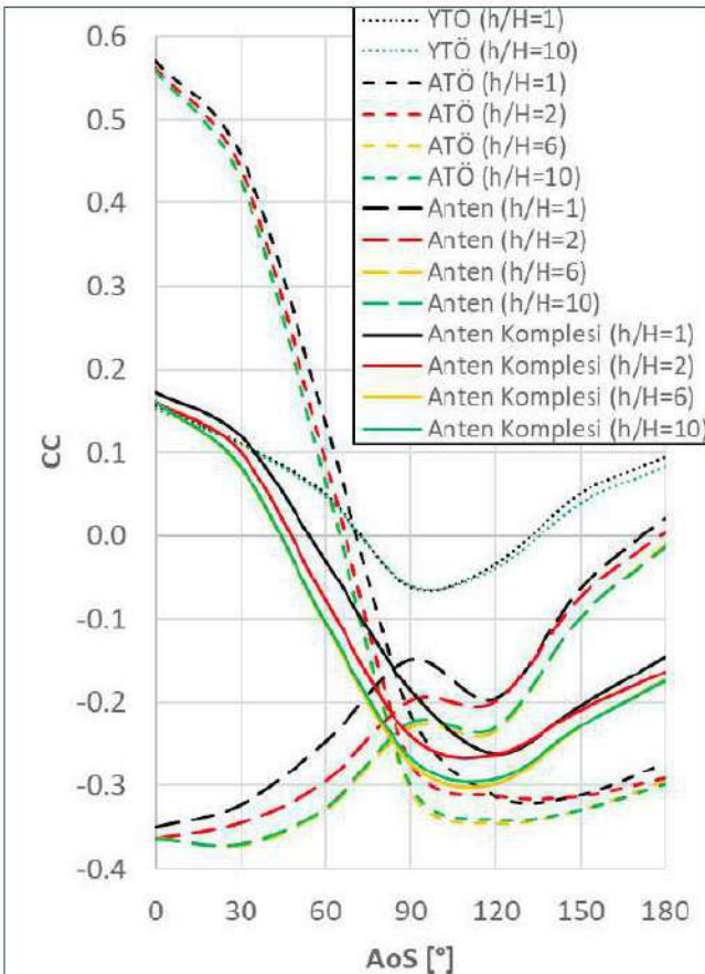
Şekil 17. Anten-Zemin Etkileşimi
