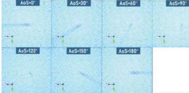
Şekil 13. Anten-Yanal Rüzgar Açısı Etkileşiminde Art-İz Kalınlıkları
