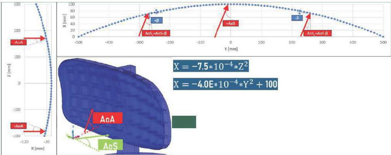
Şekil 4. Anten Geometrisini Oluşturan Eğri Denklemleri
