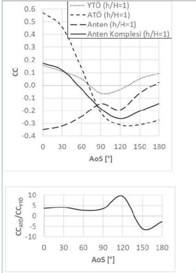
Şekil 14. Anten-Tel Örgü Etkileşimi
