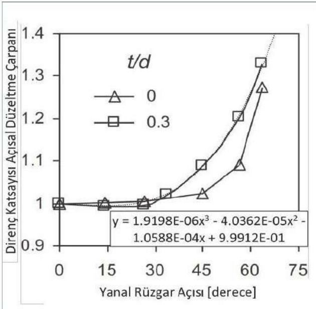
Şekil 5. Yanal Rüzgâr Açısına Göre Direnç Katsayısı Çarpanı [3]
