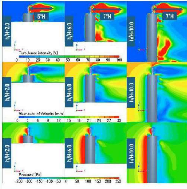
Şekil 16. Anten-Zemin Etkileşiminde Türbülans Yoğunluğu, Hız ve Basınç Alanlarının Değişimi
