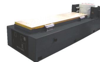
Slender slip table
